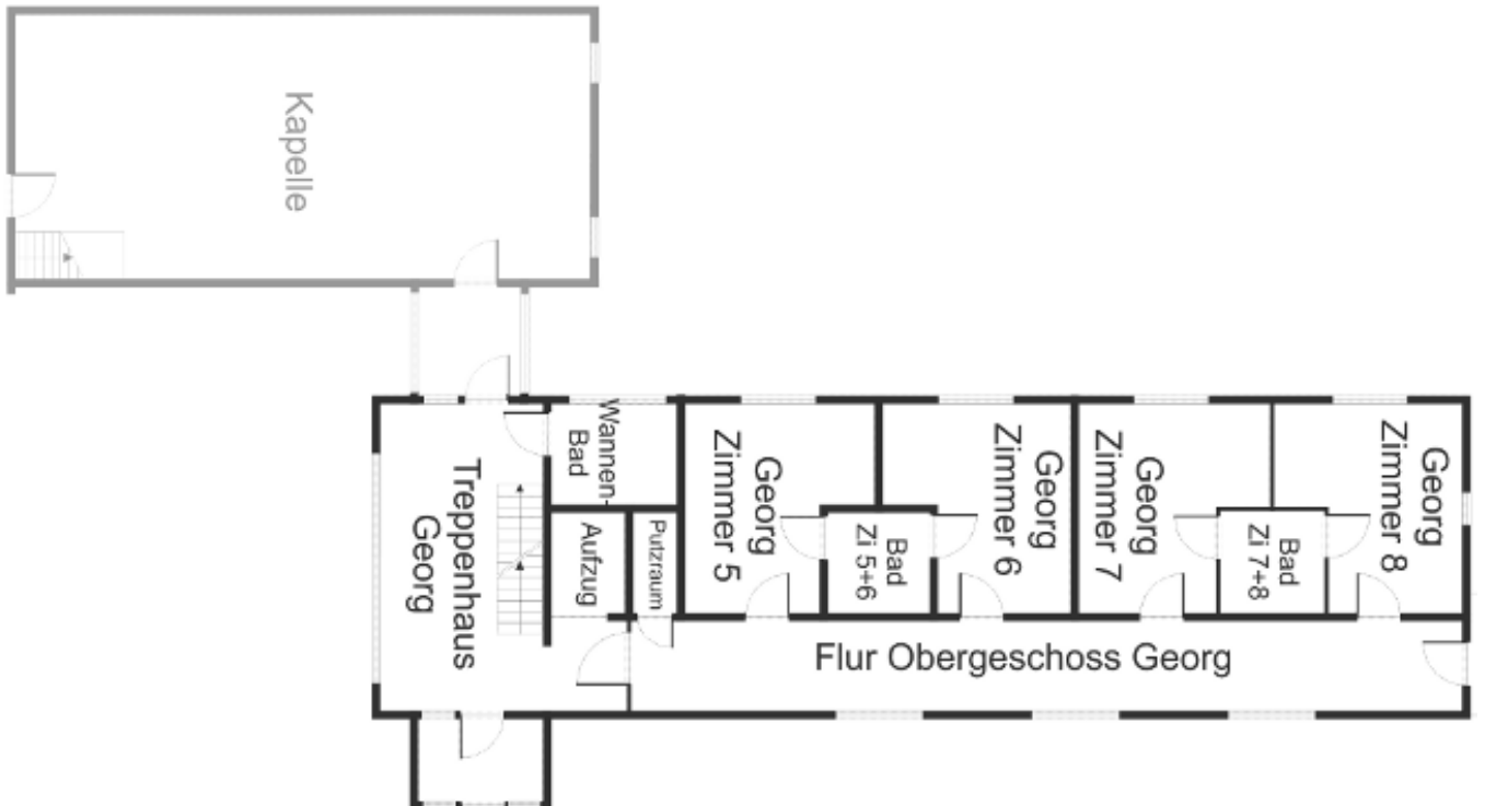
Plan des 1. Obergeschosses
